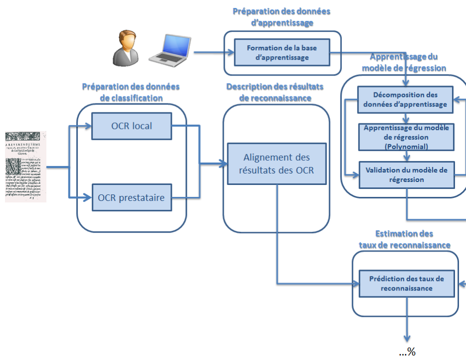
FIGURE 4.4 – Etapes des traitements de l’approche d’estimation des taux de reconnaissance de caractères qui utilise les taux moyens de désaccord
