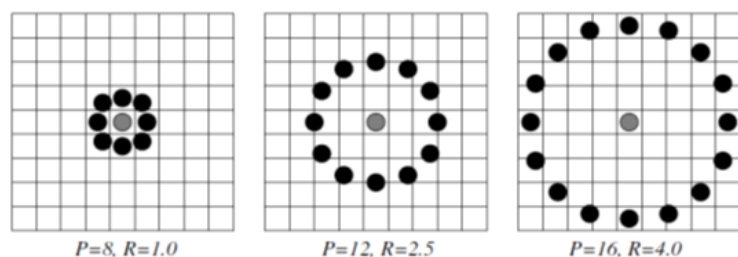
FIGURE 3.11 – L'ensemble des voisins circulaire et symétrique. Les échantillons qui ne correspondent pas à la grille des pixels sont corrigés par interpolation.
