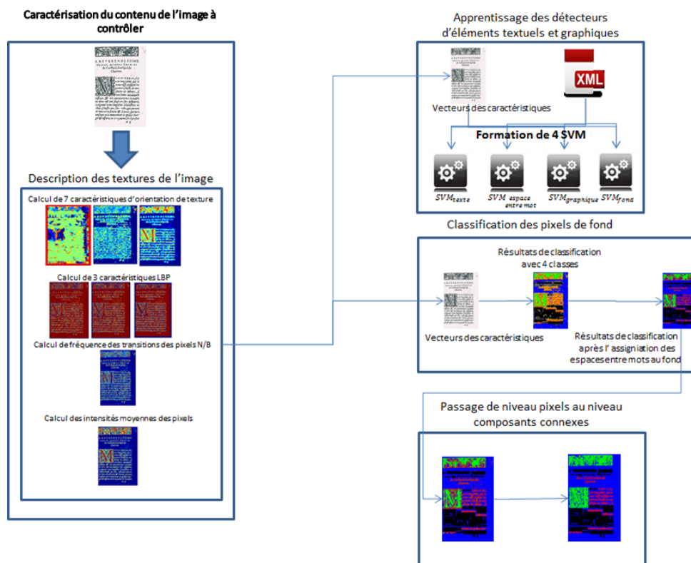
FIGURE 3.3 – Organisation des étapes de l'approche de détection des éléments omis.
