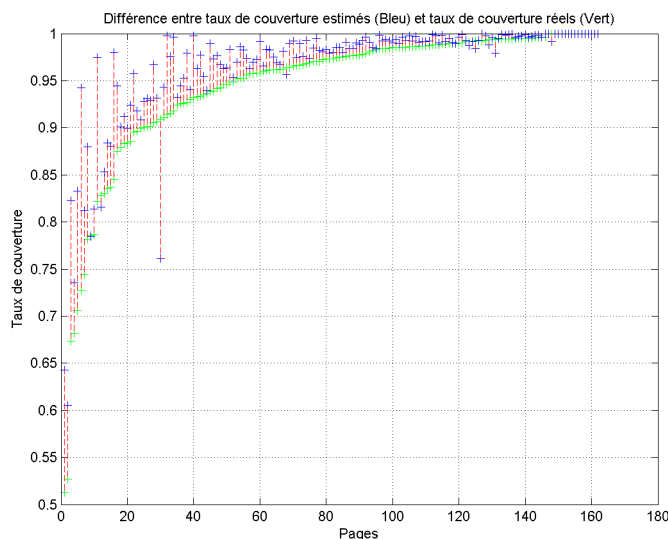
FIGURE 3.22 – Distribution simultanée des taux de couverture réels et estimés
