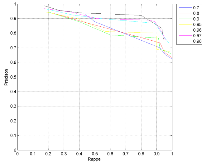
FIGURE 4.14 – Courbes rappel/précision en fonction de la valeur du seuil de rejet des documents pour le prédicteur SVR utilisant le taux de confusion entre caractères et le taux d’isogénie après une étape de sélection des documents utilisant le profil de confusion des caractères les plus fréquents (ici les trois plus fréquents)
