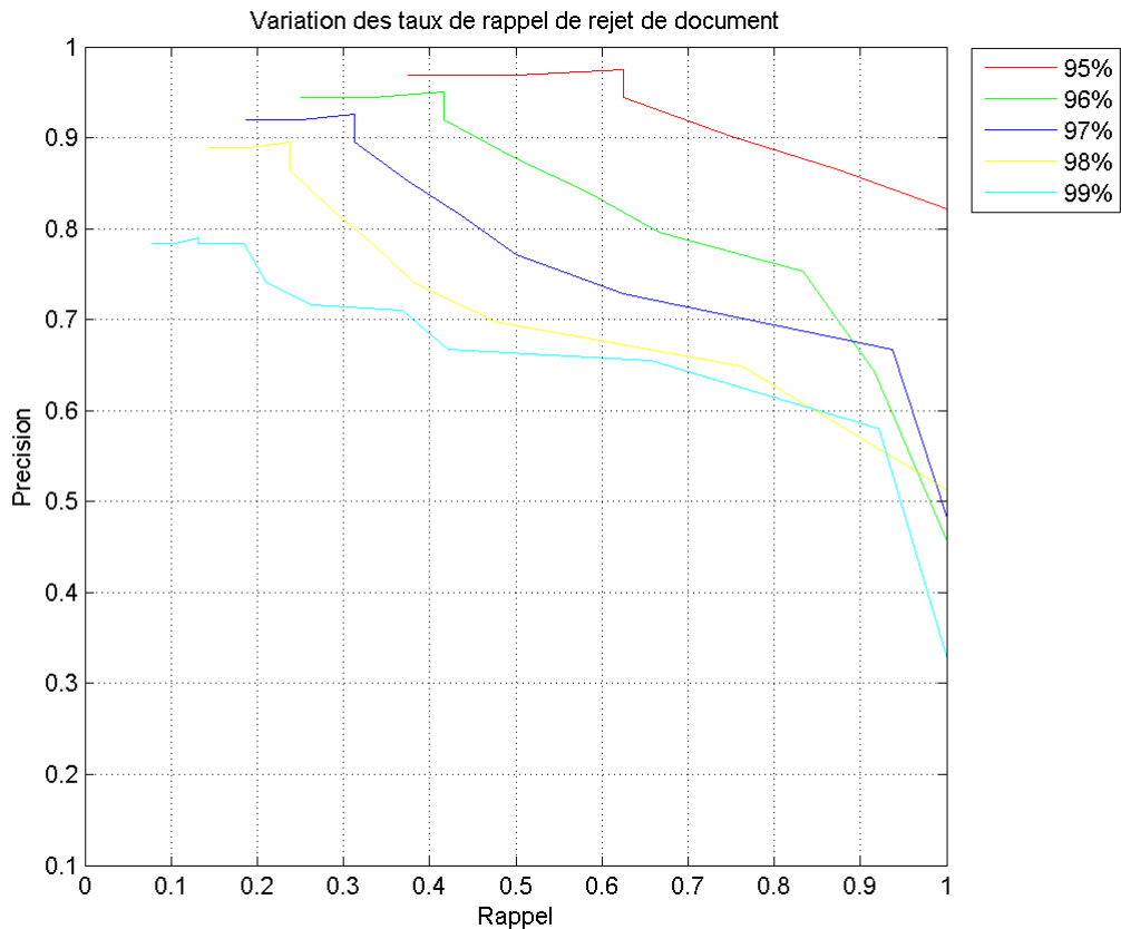
FIGURE 3.23 – Performances de notre procédure de rejet automatique des documents en variant le seuil de rejet expérimental des documents (de 80 à 99%) et pour différents niveaux de qualité exigé (seuils effectifs de 95 à 99%).
