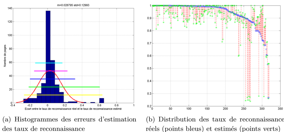
FIGURE 4.12 – Résultats de l’analyse des centiles des erreurs d’estimation obtenues avec l’approche basée sur l’utilisation simultanée des données d’isogénie et d’alignement des résultats d’OCR
