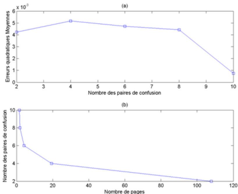
FIGURE 4.7 – Variation de l’erreur quadratique moyenne et du nombre des pages d’apprentissage en fonction du nombre des paires de désaccord qui constituent la signature de la page.
