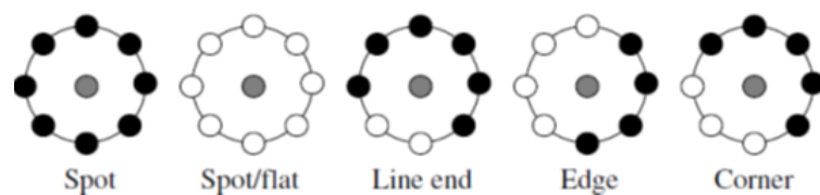
FIGURE 3.12 – Exemples de motifs locaux détectés par le descripteur LBP
