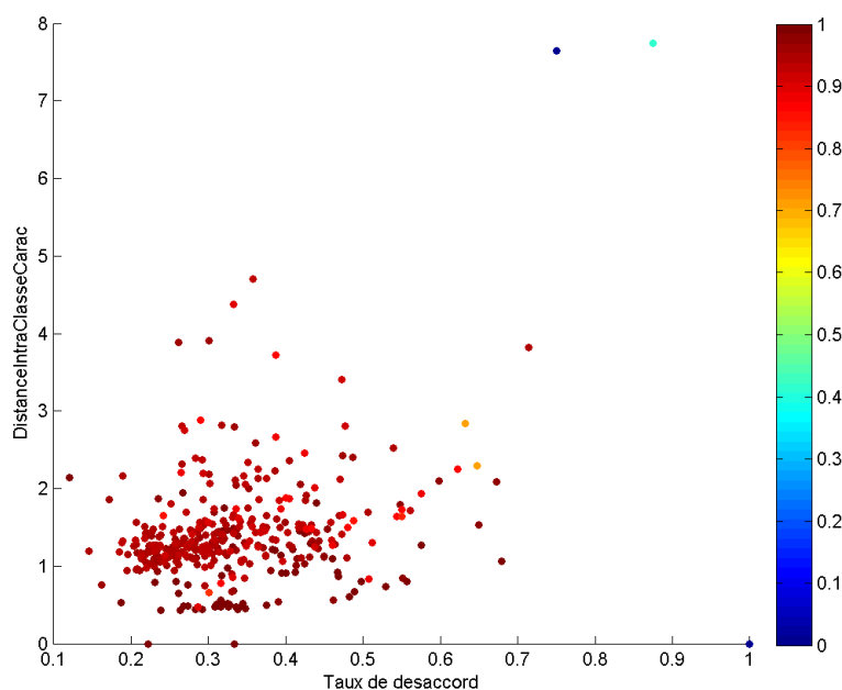
FIGURE 4.6 – Distribution de 230 pages tirées de façon aléatoire en fonction des taux de désaccord et des distances intra-classe de caractère. Les points rouges correspondent aux pages ayant des forts taux de reconnaissance. Les points bleus correspondent aux pages ayant des faibles taux de reconnaissance.
