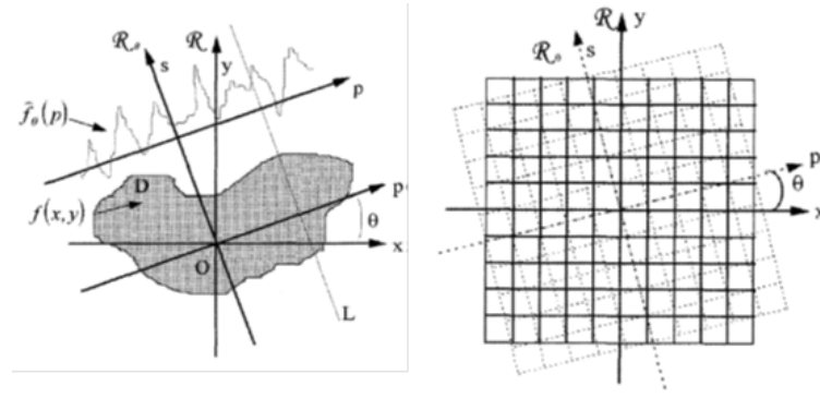
FIGURE 3.5 – Représentation de la transformée de Radon. L'image à gauche représente la projection f_{\Theta}(p) de l'image définie dans le repère en rotation.
