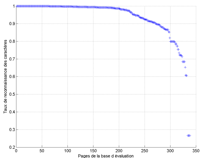
FIGURE 4.8 – Distribution des taux de reconnaissance des caractères de la base des documents d'évaluation
