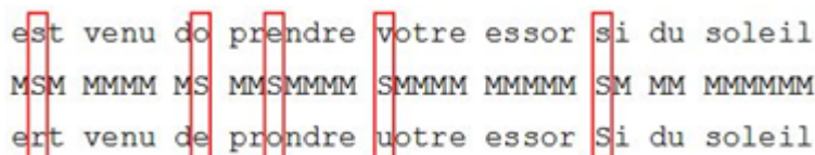
FIGURE 4.3 – Un exemple de résultat d’alignement des caractères des mots de l’OCR des prestataires (en haut) avec les caractères des mots de l’OCR de validation (en bas). Au milieu, les opérations d’éditions nécessaires (M=matching ; S=Substitution ; D=suppression). Les cadres rouges représentent les caractères en désaccord entre deux OCR.
