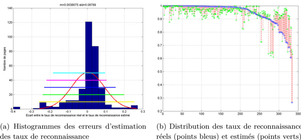
FIGURE 4.11 – Résultats de l'estimateur basé sur les données d'alignement des résultats d'OCR
