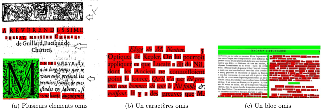
FIGURE 3.1 – Exemples des résultats d’OCR fournis par des prestataires ; les rectangles rouges représentent les boîtes englobantes des mots, le rectangle vert qui délimite la lettrine représente l’élément graphique ; (a) Exemple de résultat d’OCR qui regroupe des mots partiellement détectés, des mots entièrement omis et des illustrations complètement oubliées. (b) Exemple de caractère manquant dans les résultats d’OCR, (c) Exemple d’un résultat d’OCR avec omission d’un bloc textuel et confusion d’un bloc de texte en graphique.
