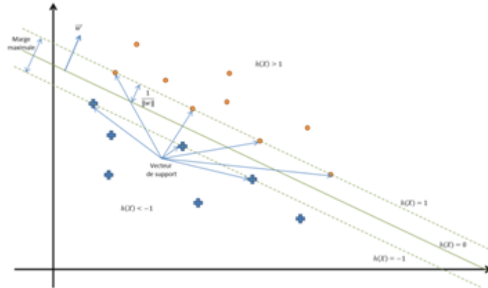
FIGURE 3.16 – L’hyperplan optimal séparant la classe des plus des classe des cercles
