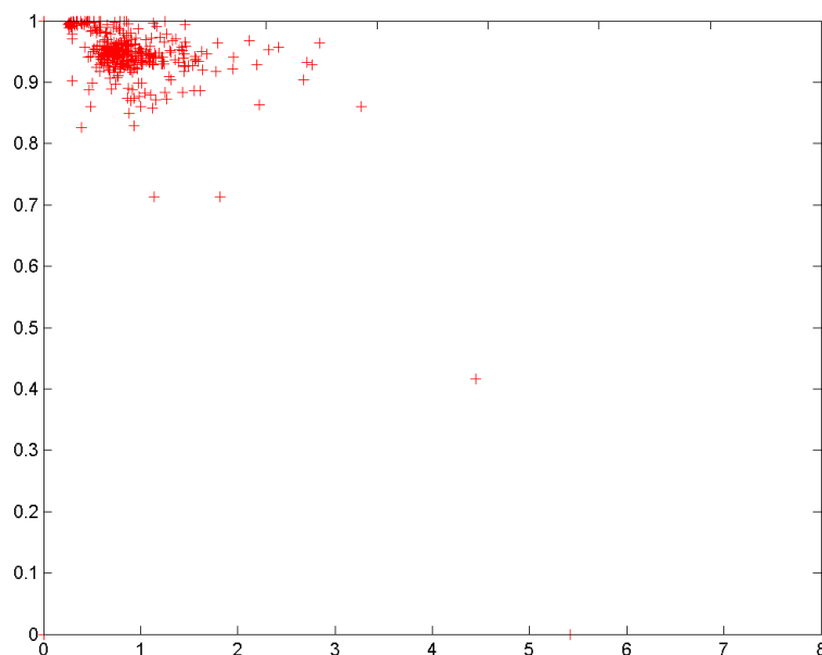
FIGURE 4.2 – Représentation de 230 pages selon le taux de reconnaissance des caractères et la distance moyenne intra-classe de caractères. L’axe d’abscisse représente les distances moyennes intra-classes de caractères, l’axe des ordonnées représente des taux de désaccord.
