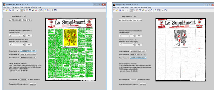
FIGURE 3.24 – Interface graphique : détection sur une image (gauche) et même image avec zones masquées (droite).
