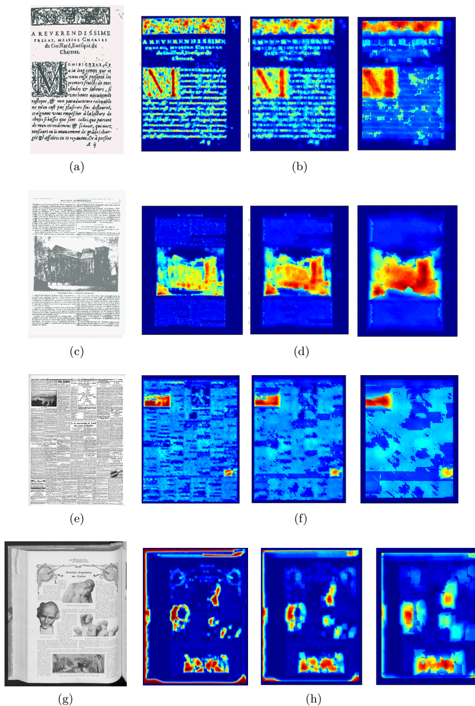
FIGURE 3.9 – Réponses de descripteur f_{(k+1)} qui utilise l'intensité médiane des orientations de texture pour décrire les régions de la page.
