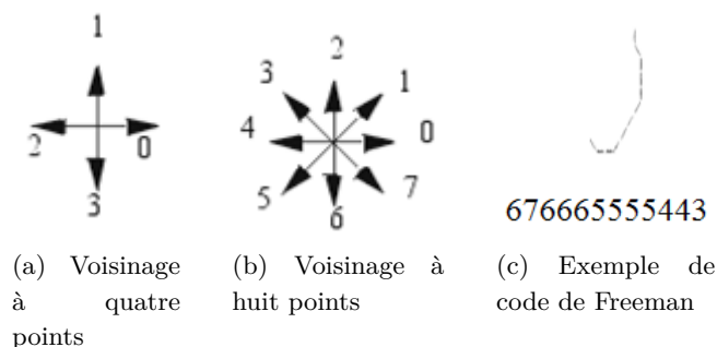
FIGURE 2.4 – Exemple de Code de Freeman obtenu sur le squelette de caractère arabe , le point de départ est le point supérieur de forme.
