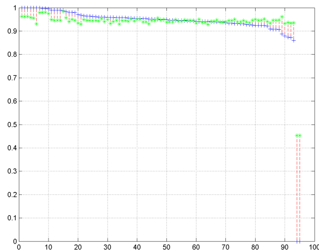
FIGURE 4.10 – Résultats de l'estimateur basé sur les données d'isogénie sur une base d'images homogène
