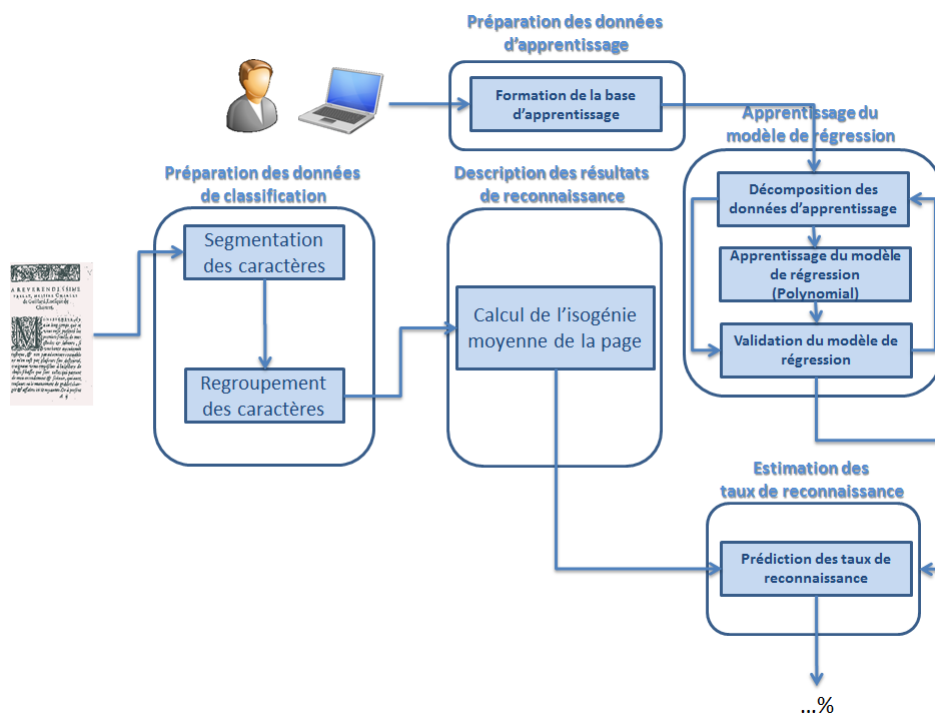
FIGURE 4.1 – Etapes des traitements de l’approche d’estimation des taux de reconnaissance de caractère qui utilisent les distances intraclasse de caractère
